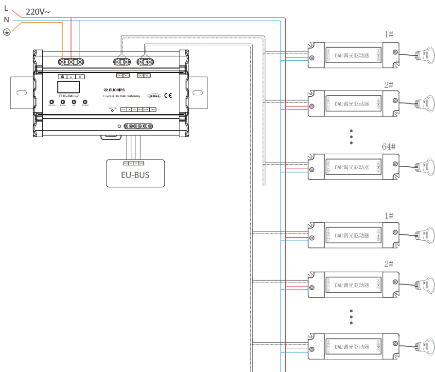
应用连接图
