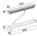
Wallwasher ad incasso con lenti L. 620 / Recessed Wallwasher with lens L. 620
