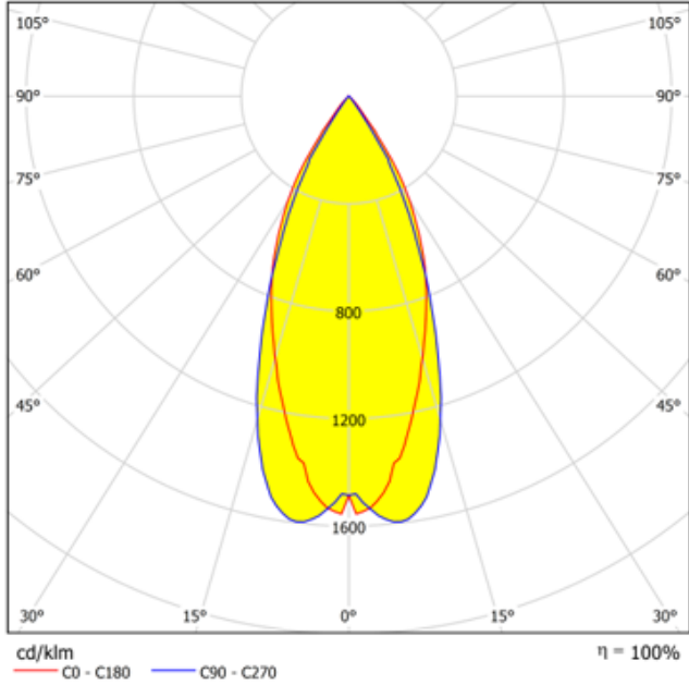
38° Black Baffle Glare
