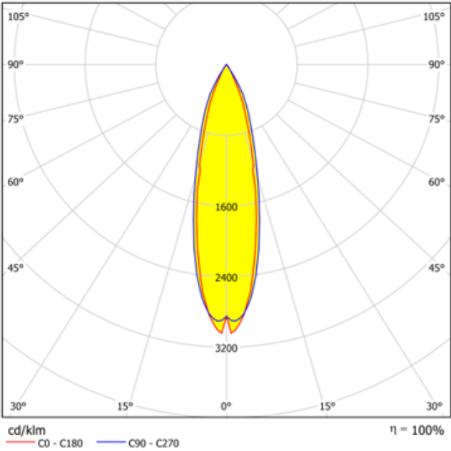
27° Black Baffle Glare
